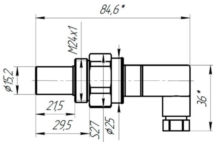
Рис.3. Установочные и габаритные размеры преобразователя DW2TC-B.
