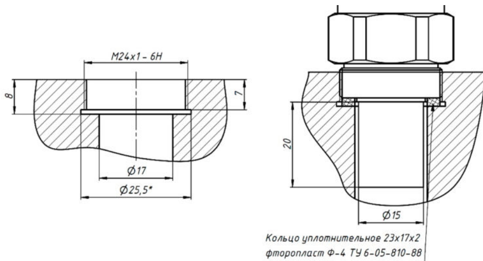
Рис.4. Конструкция фланца для подключения измерительного преобразователя ДВ2ТС-В к газовой магистрали.
